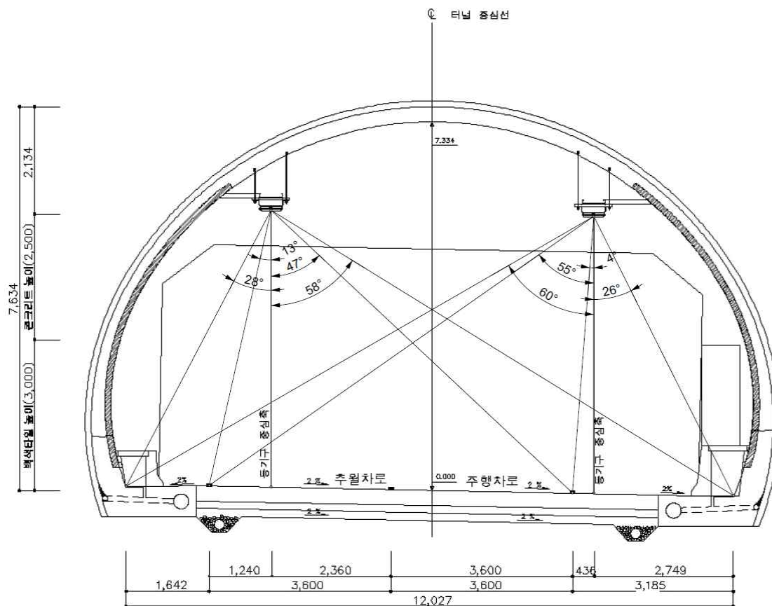
부록-〈그림 2.4〉 터널의 단면도
