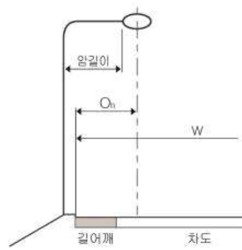
(b) 길어깨가 좁을 경우
