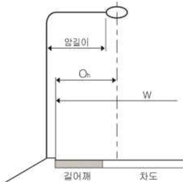
(a) 길어깨가 넓은 경우
