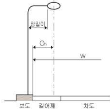
(d) 보도가 좁을 경우
