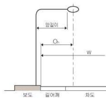
(c) 보도가 넓은 경우
