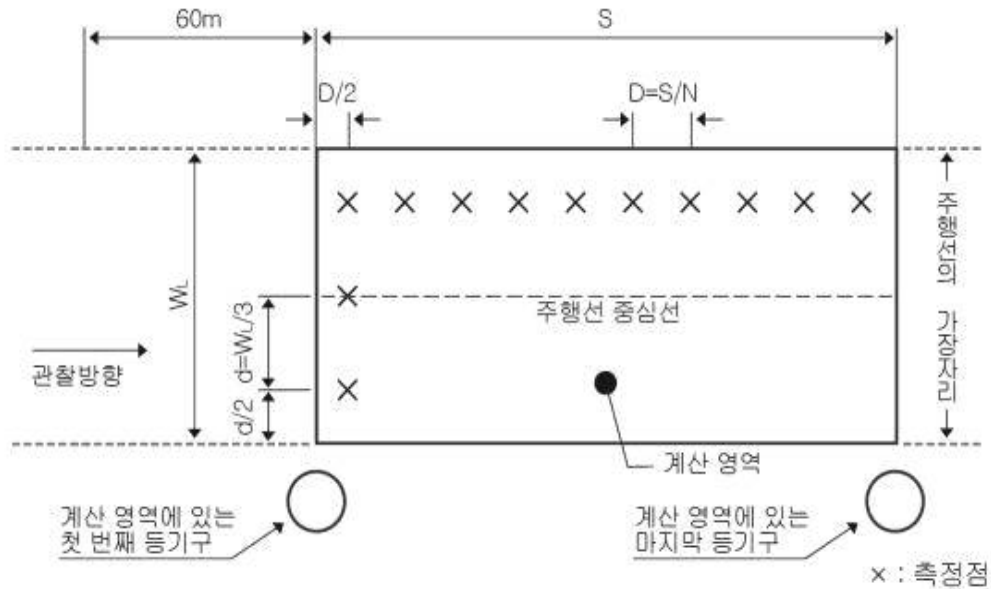
부록-〈그림 4.3〉 주행선에서 측정점의 위치
