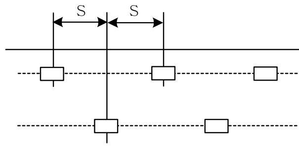
(b) 지그재그 배열
